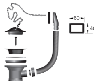
Bottenventil UTAN / MED bräddavlopp RSK 808 65 47 RSK 808 65 45
