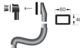
Bottenventil UTAN / MED bräddavlopp RSK 808 65 47 RSK 808 65 45
