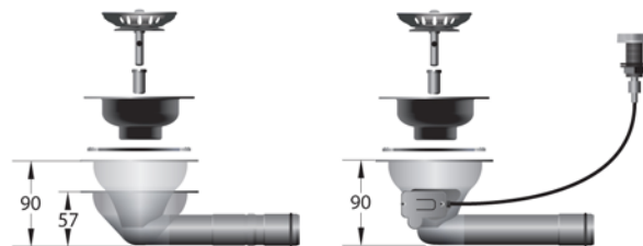
Korgventil 90° LÅG / HÖG RSK 808 65 59 (Låg 57) RSK 808 65 58 (Hög 90)
